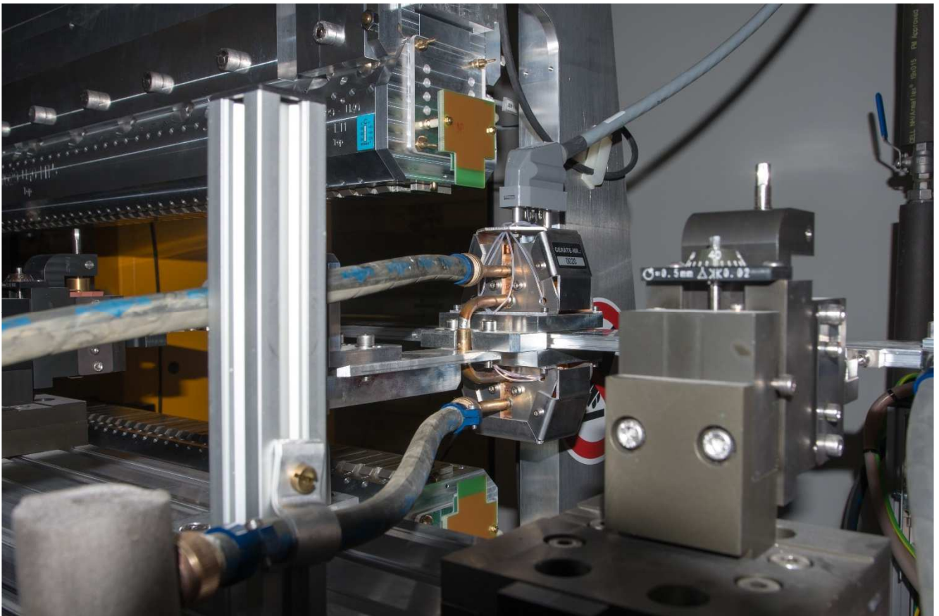
Ansicht Frontseite des Undulators mit je einer Radfetteplatte Oben und Unten. Dienstag, 9. März 2021
