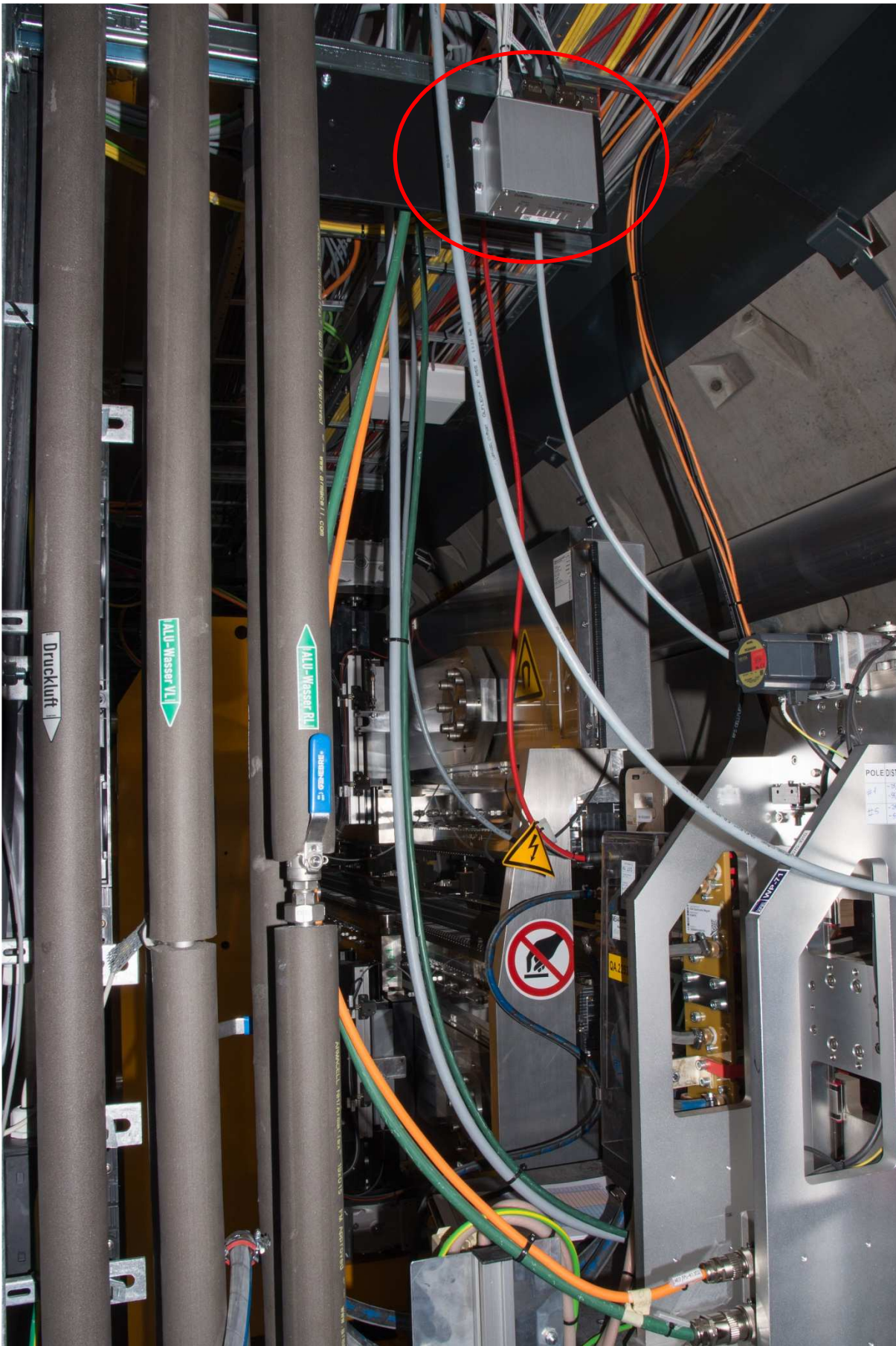
DosiBox auf schwarzer HDPE-Grundplatte an Hilti Konsole montiert.
