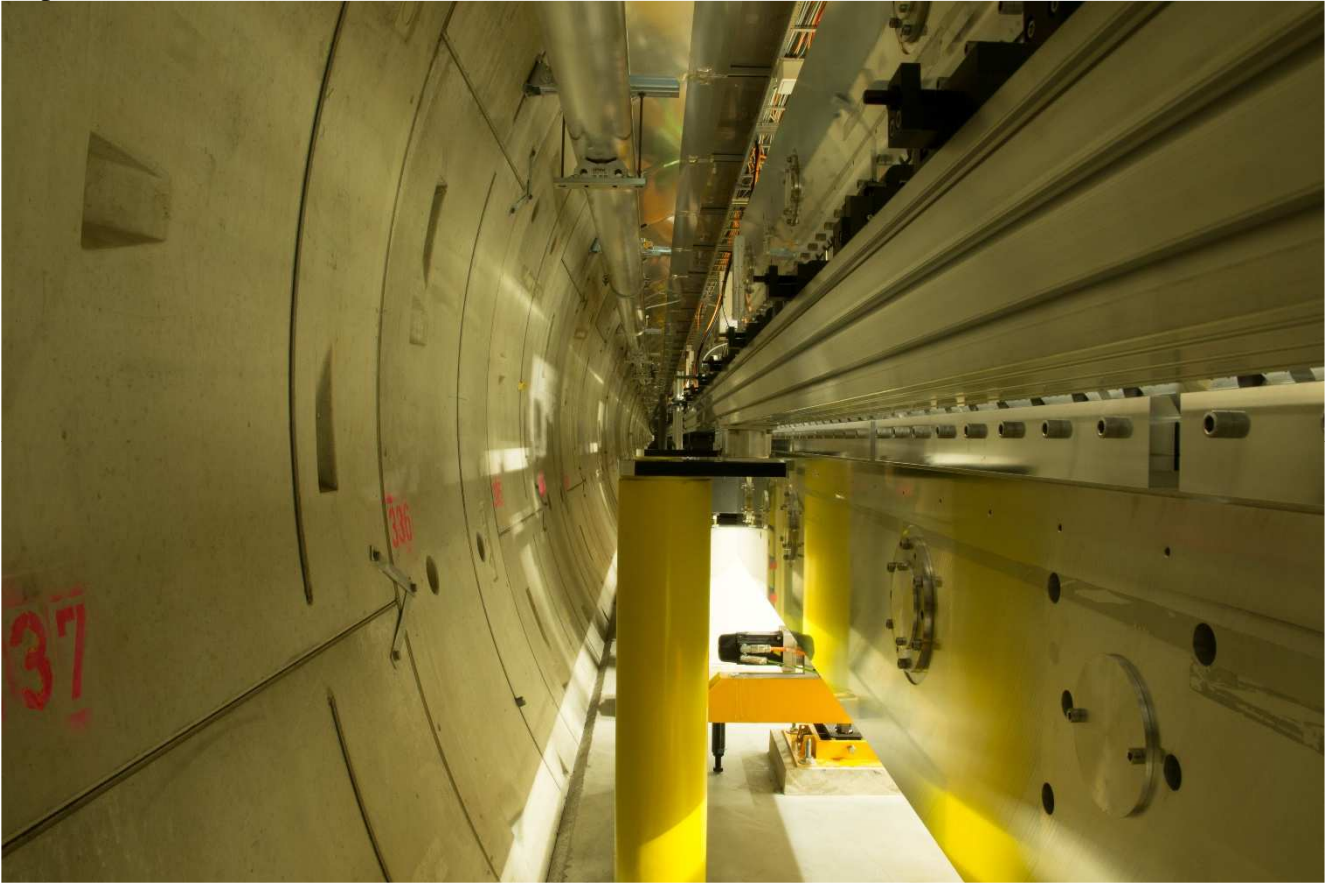
Ansicht Rückseite Undulator in Strahlrichtung.
