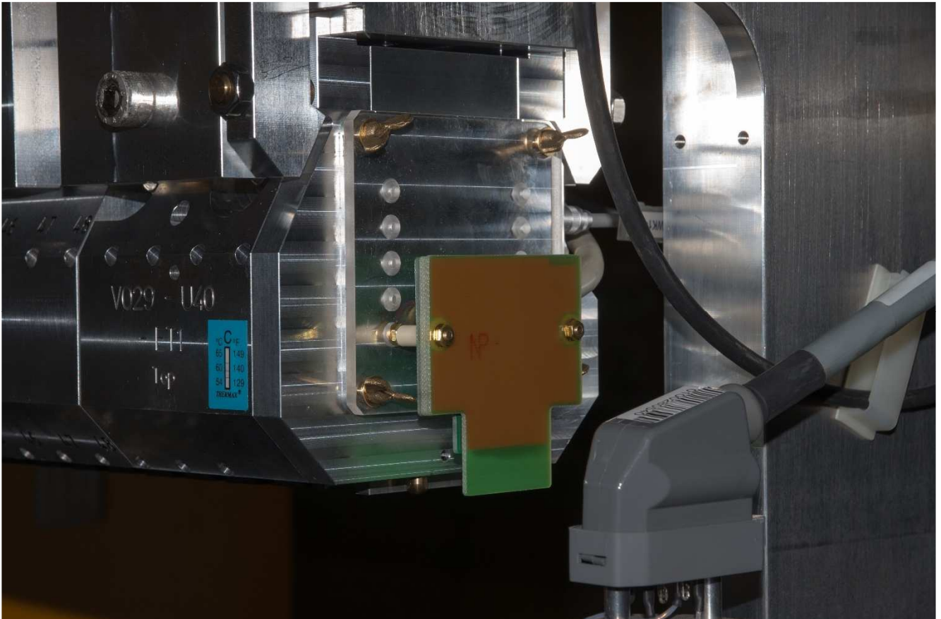
Radfetteplatte Oben an Frontseite des Undulators. Blickrichtung Gang.
