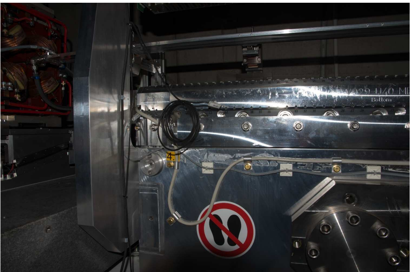
Leitungsführung der Radfetplatine Unten. Im Hintergrund die Tunnelwand.
