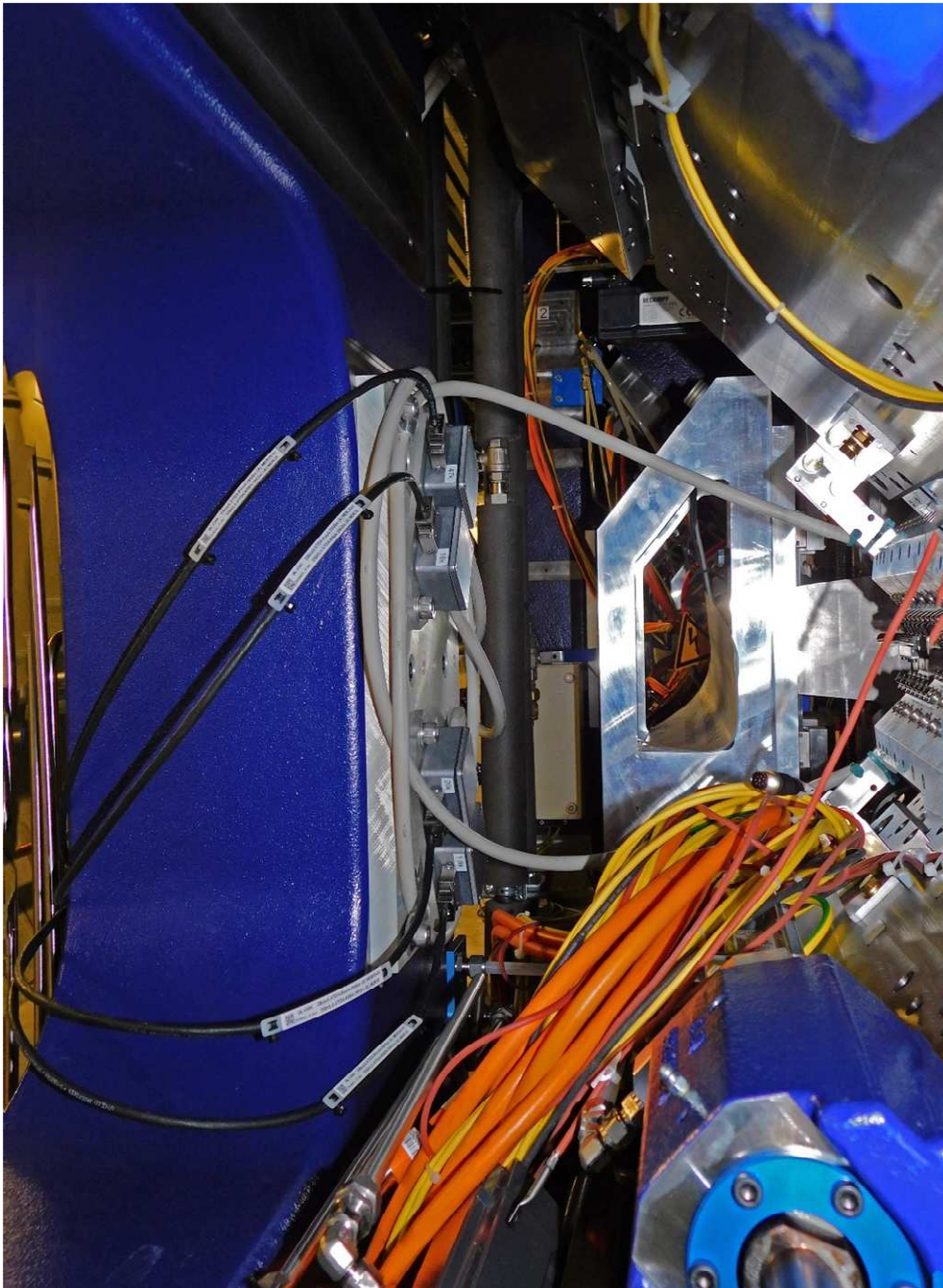
Rückseitige Ansicht der vier montierten Übox-Gehäuse mit MDR-Kabel.
