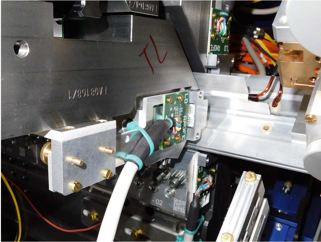
Vorderansicht Montage RadFet
