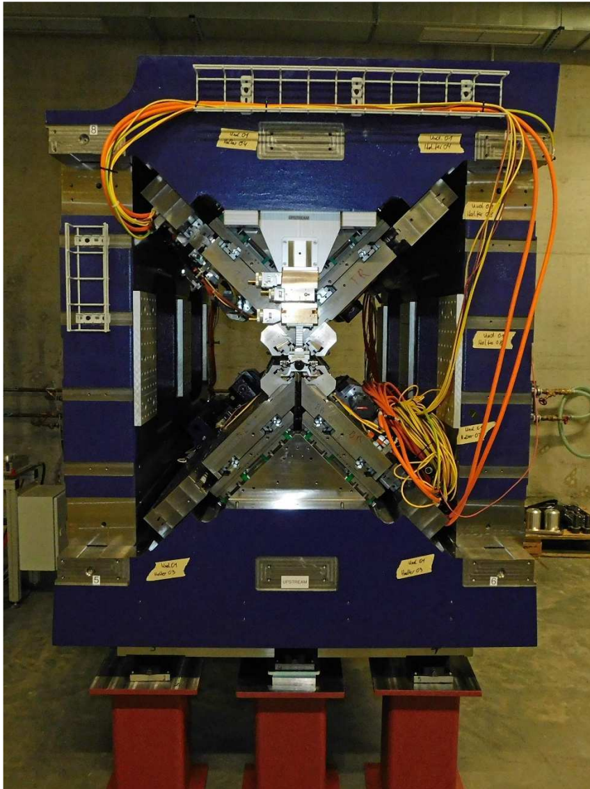
Frontansicht/Upstream
