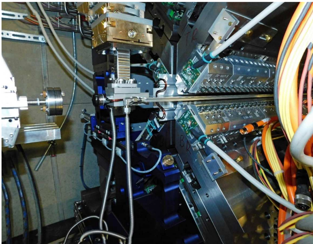
Einbau von vier RadFet-Platinen mit Halterung in Strahlrichtung/Upstream.
