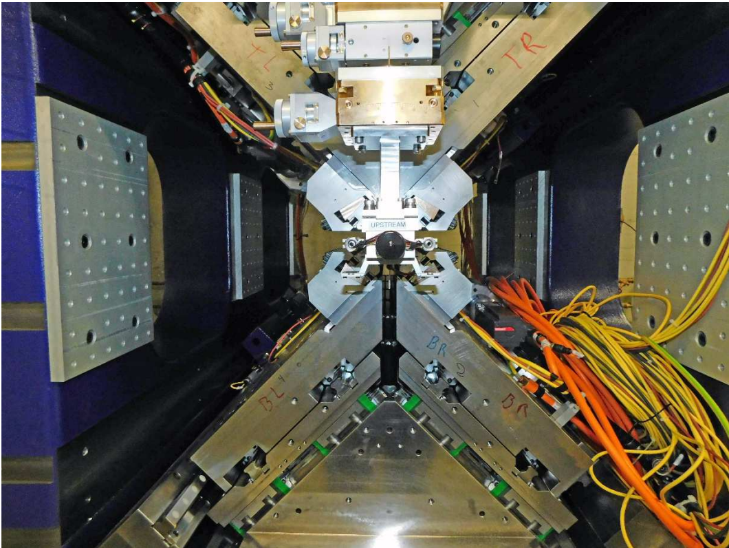
Frontansicht/Upstream
