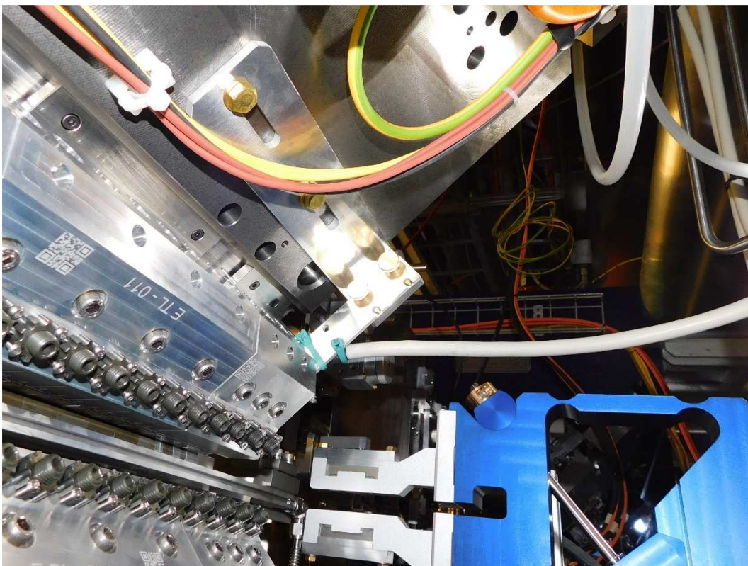
Rückansicht Montage RadFet
